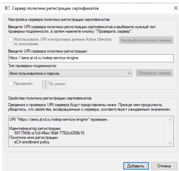
Рисунок 54 – Проверка сервера выполнена успешно
