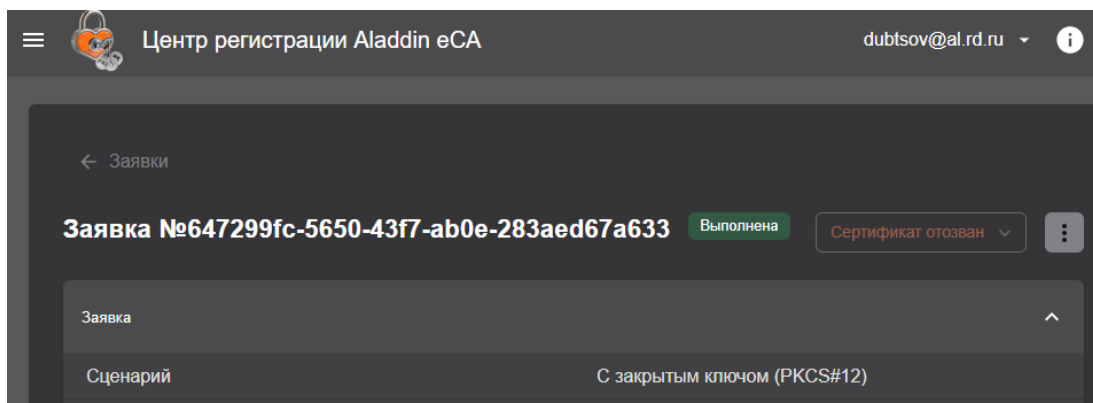
Рисунок 47 – Сертификат отозван
