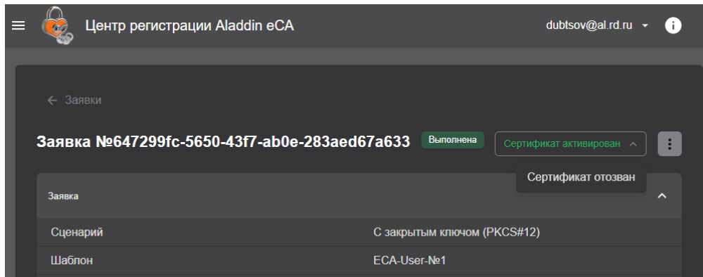
Рисунок 45 – Отзыв сертификата
