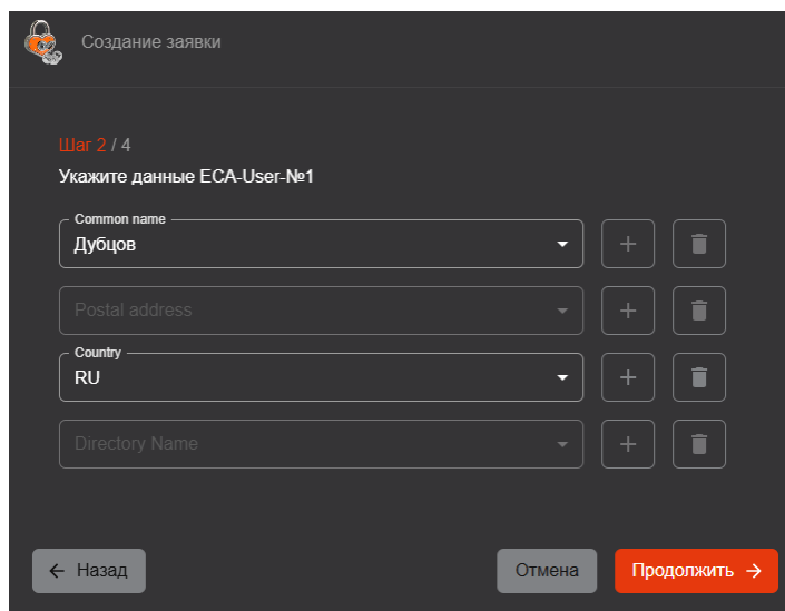
Рисунок 28 – У получателя сертификатов (субъекта PC) отсутствуют необязательные по шаблону атрибуты
