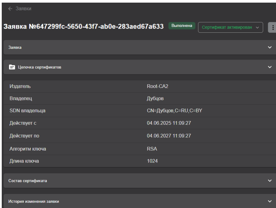
Рисунок 17 – Карточка заявки, по которой выпущен сертификат
