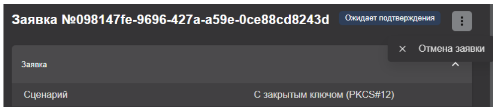
Рисунок 40 – Инициализация процесса отмены заявки на выпуск сертификата из ее карточки
