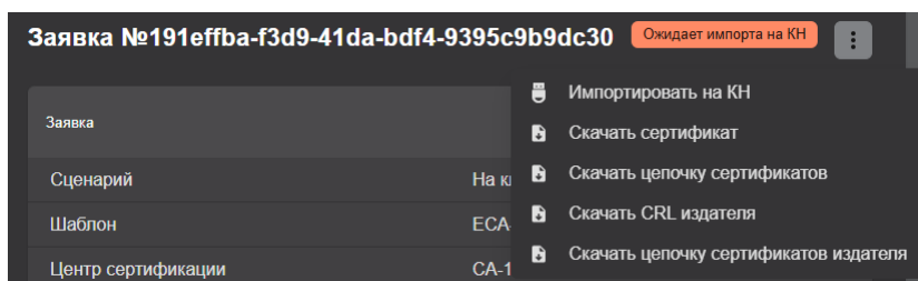
Рисунок 49 – Инициализация процесса импорта сертификата на ключевой носитель из карточки заявки
