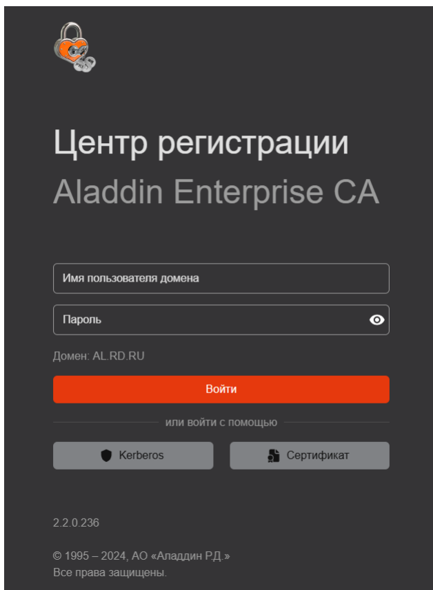
Рисунок 2 – Окно авторизации
