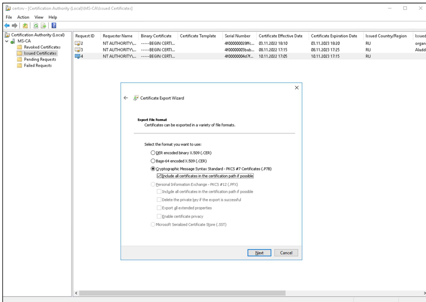
Рисунок 13 – Окно экспорта цепочки сертификатов
