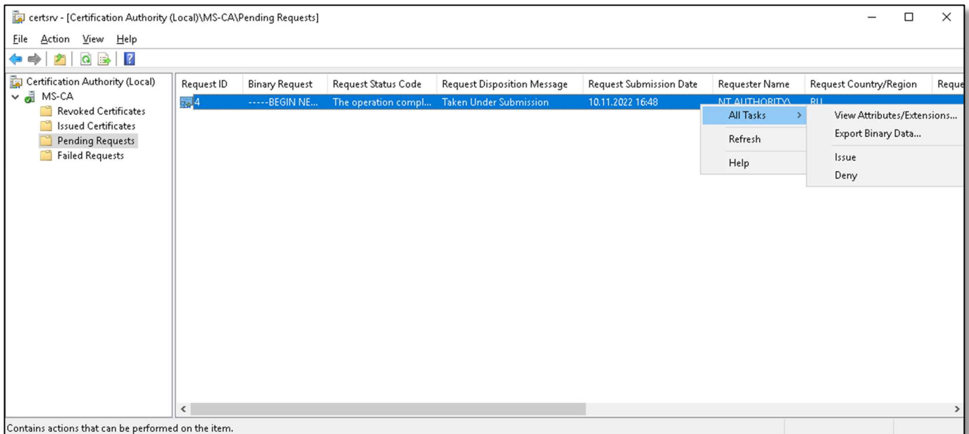
Рисунок 11 – Окно запросов в ожидании Центра сертификации
