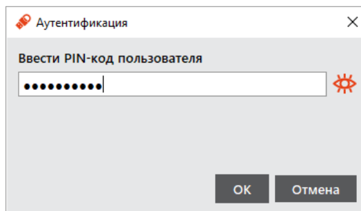
Рисунок 49 – Окно "Аутентификация"
