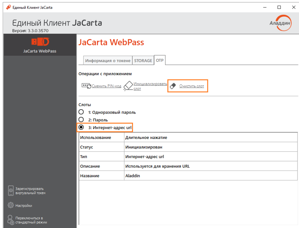
Рисунок 85 – Очистка слота
